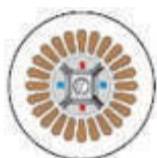
Сосредоточенные обмотки
